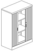
ZA-0913 W900 x D470 x H1320 ZA-1013 W1000 x D470 x H1320 ZA-1213 W1200 x D470 x H1320
