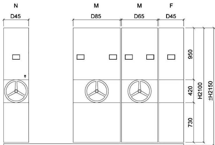
側視圖
