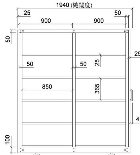
正視圖
