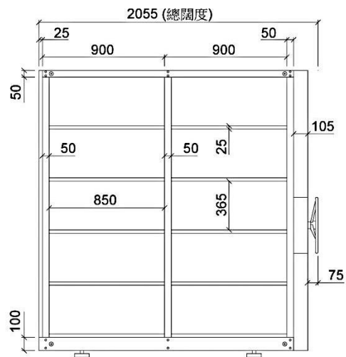
正視圖
